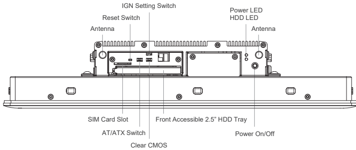
Left I/O
