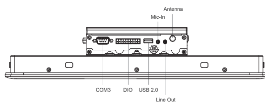
Right I/O
