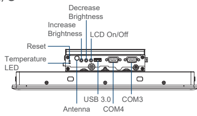
Left I/O
