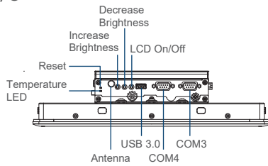
Left I/O
