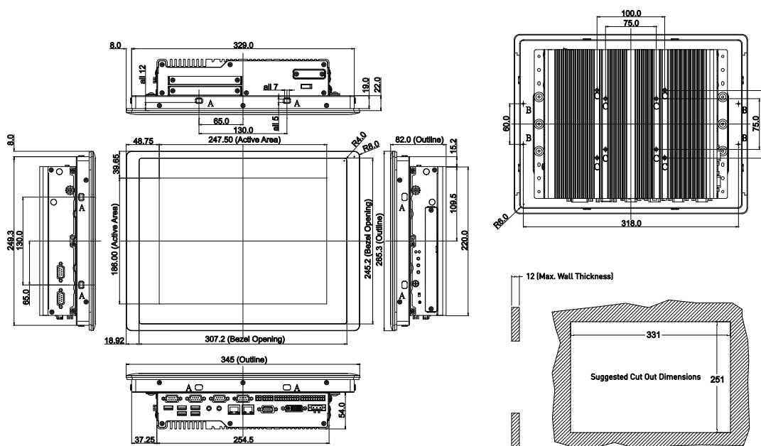
CS-112H/P2002
