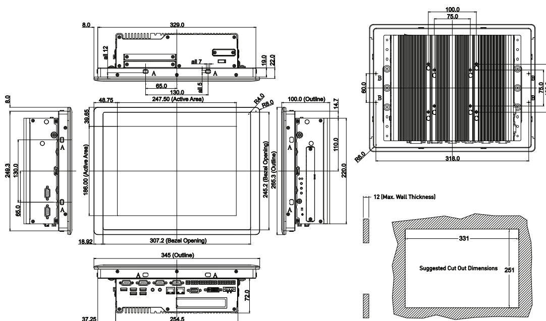
CS-112H/P2002E
