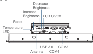
Left I/O
