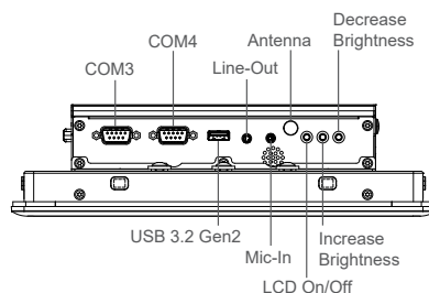
Right I/O
