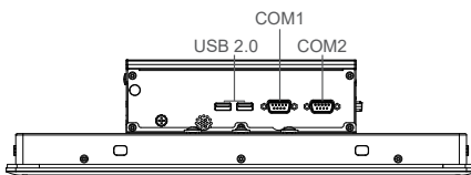
Left I/O
