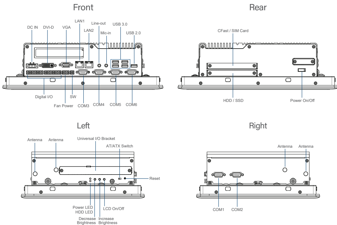
CS-117/P2002E
