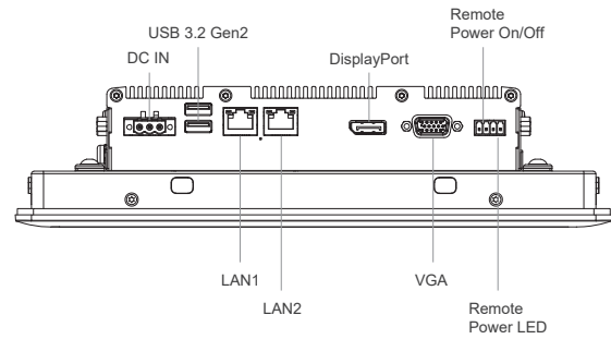
Right I/O
