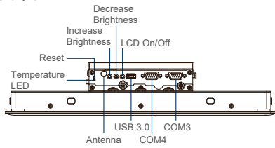
Left I/O
