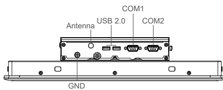
Left I/O
