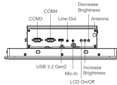
Right I/O
