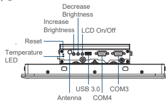
Left I/O
