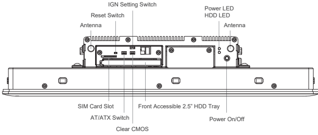
Left I/O
