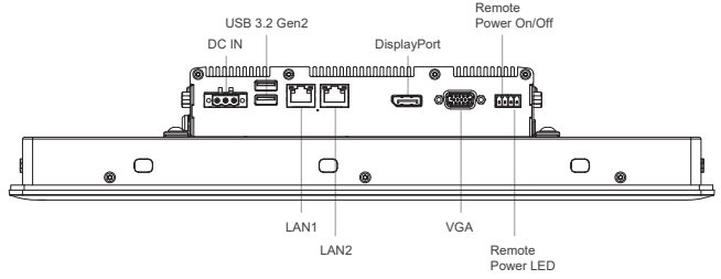
Right I/O
