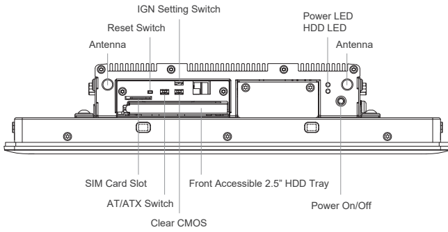
Left I/O
