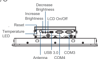
Left I/O
