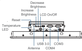
Left I/O
