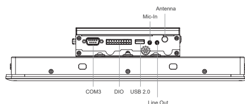
Right I/O
