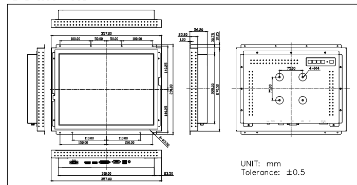
OPD-1156A RS232
