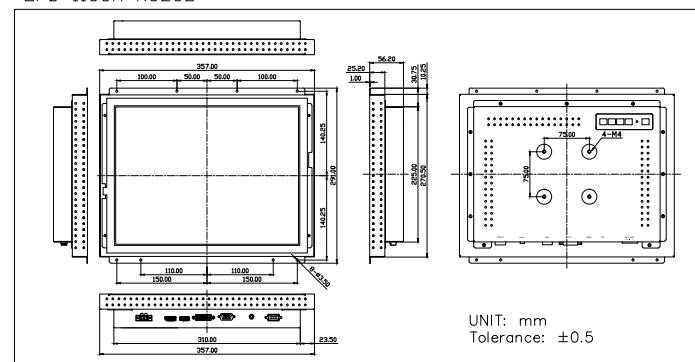
OPD-1156A RS232
